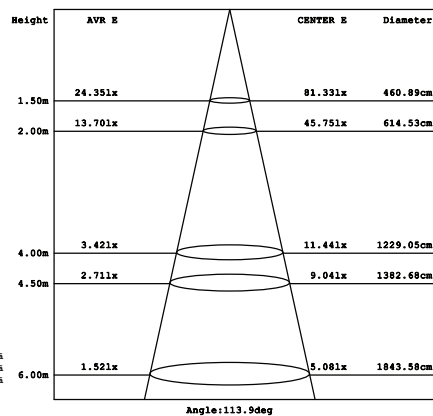
Parameter of PL-R06 | CCT 4000K
