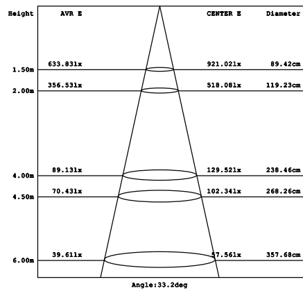
Parameter of DL-HW1x10 | CCT 4000K
