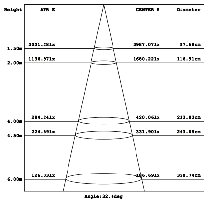
Parameter of DL-HW2x15 | CCT 4000K
