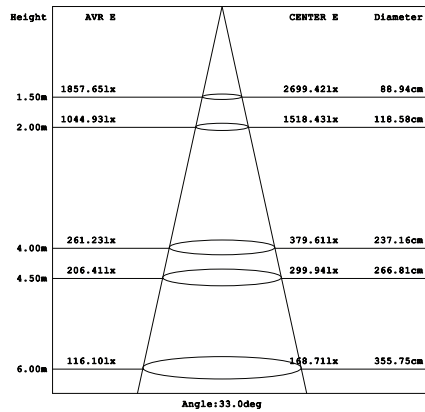
Parameter of DL-HW3x10 | CCT 4000K
