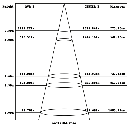
Parameter of HB-DS90 | CCT 4000K
