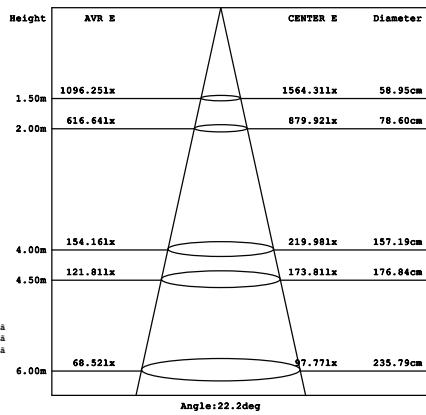
Parameter of OS-DG13 | CCT 4000K
