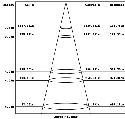
Parameter of CL-CW30/ CL-CB30 CCT 4000K
