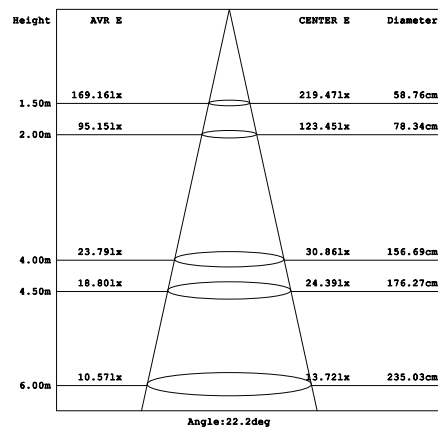
Parameter of DL-DW3 | CCT 4000K
