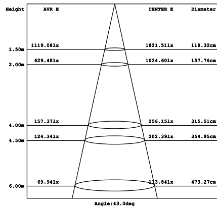
Parameter of DL-GW25 | CCT 4000K
