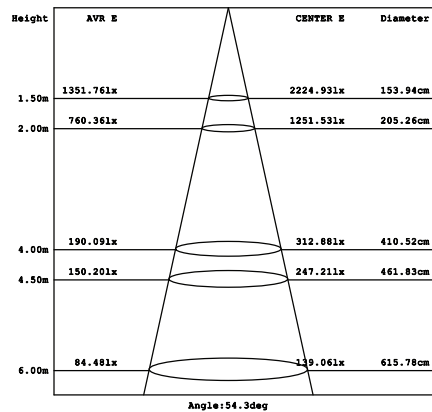
Parameter of DL-GW35 | CCT 4000K
