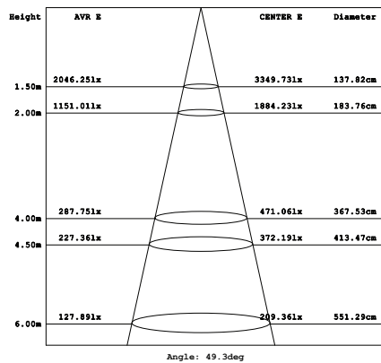
Parameter of DL-GW50N | CCT 4000K
