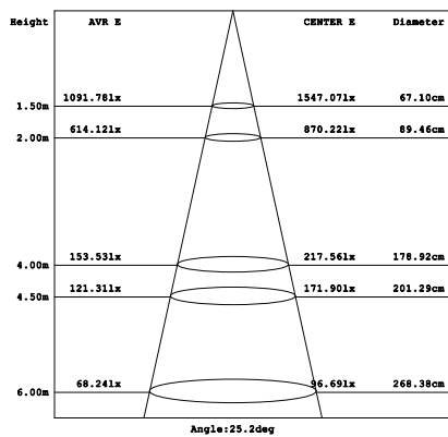
Parameter of DL-IW10 | CCT 4000K
