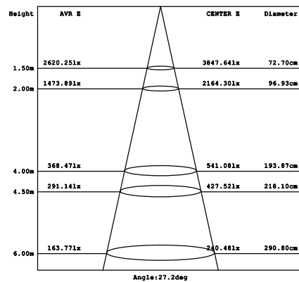
Parameter of DL-IW30 | CCT 4000K
