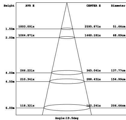
Parameter of DL-NW14 | CCT 4000K
