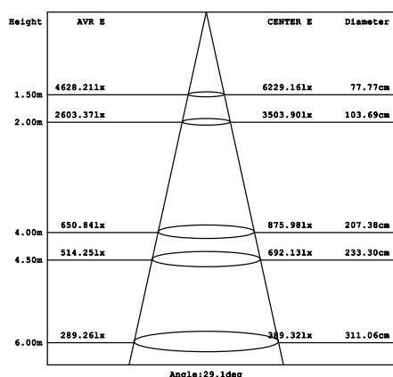
Parameter of DL-PW50/ DL-PB50 | CCT 4000K
