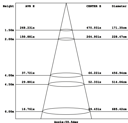
Parameter of DL-RW10 | CCT 4000K
