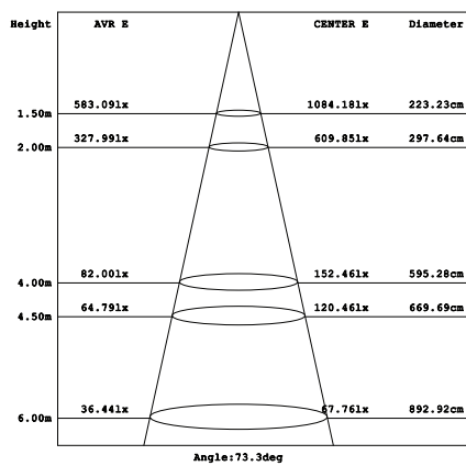
Parameter of DL-JW30 | CCT 4000K
