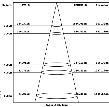
Parameter of GS-AW60 | CCT 4000K
