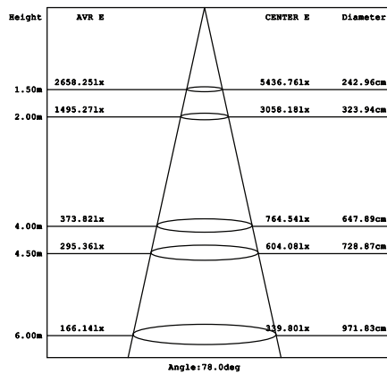
Parameter of GS-CW140 | CCT 3000K
