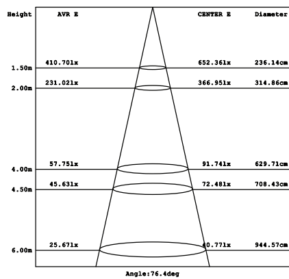
Parameter of ST-AG60 CCT 4000K
