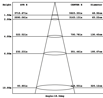
Parameter of TR-JW25 | CCT 4000K
