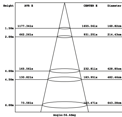
Parameter of TR-KW35/TR-KB35 | CCT 4000K
