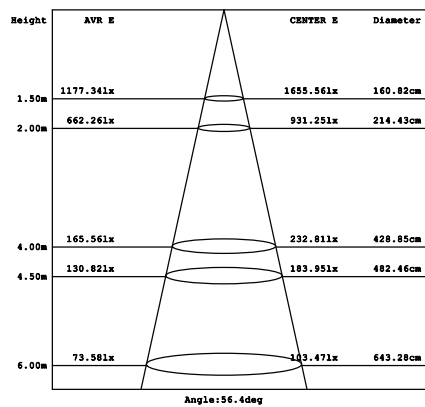
Parameter of TR-LW35/TR-LB35 | CCT 4000K
