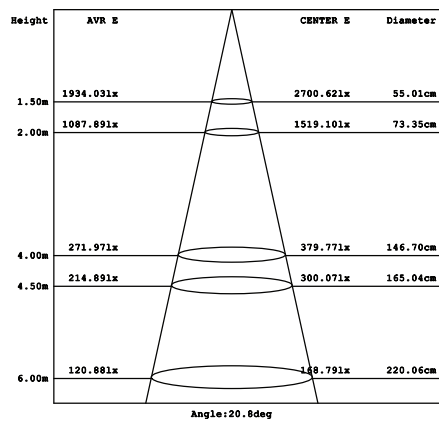
Parameter of UW-CS12 | CCT 4000K
